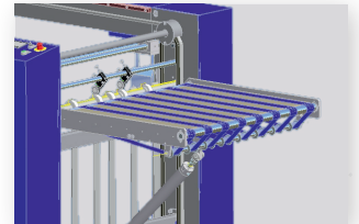
Klappbarer Transporttisch
