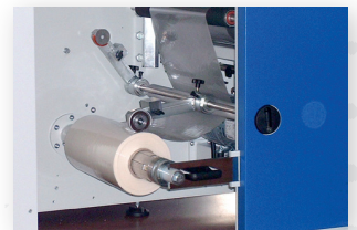
Zweite Folieneinrichtung
