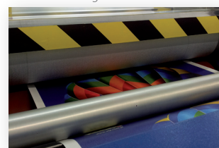
Hochwertiges embossieren durch gelaserte Walze
