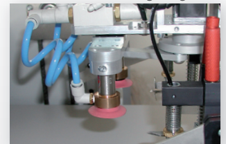
Prozesssicherer Sauganleger
